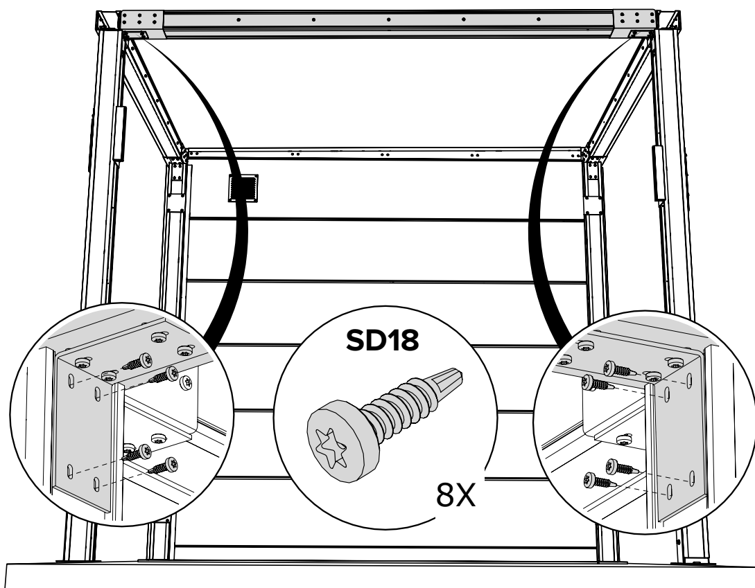
I Fachada / Fachada
