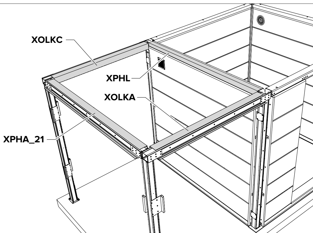
H+I+J Fachada / Fachada
