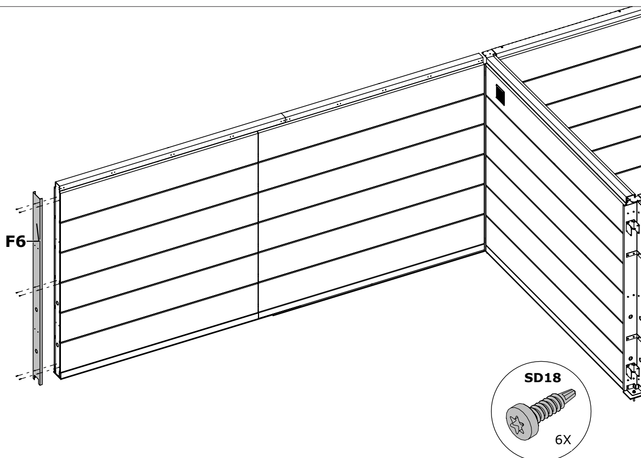
H Fachada / Fachada
