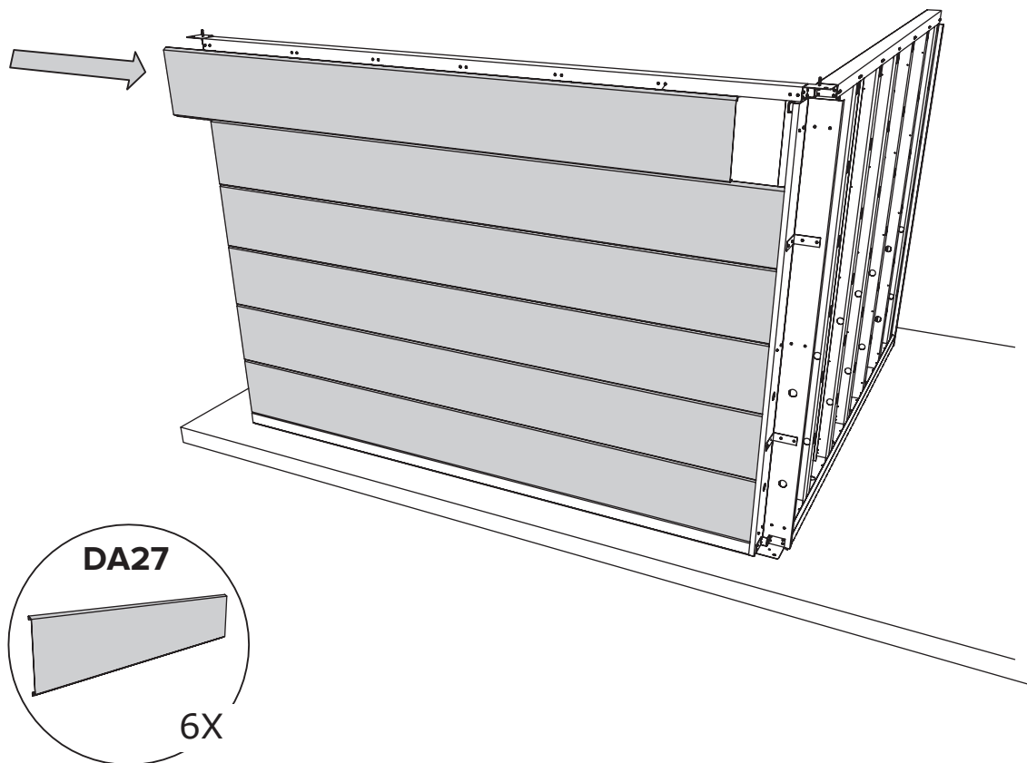
C + D Fachada / Fachada
