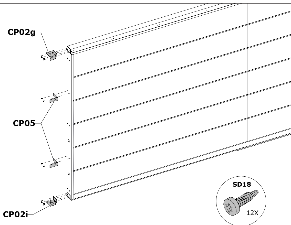
H Fachada / Fachada
