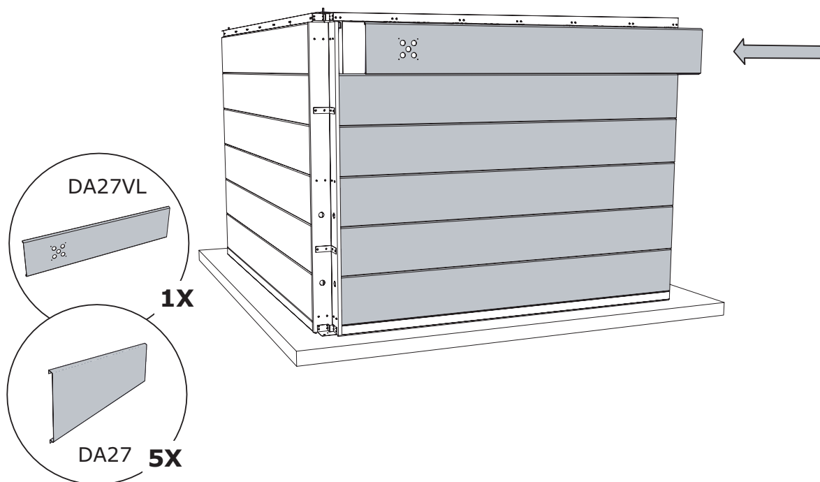
C + D Fachada / Fachada
