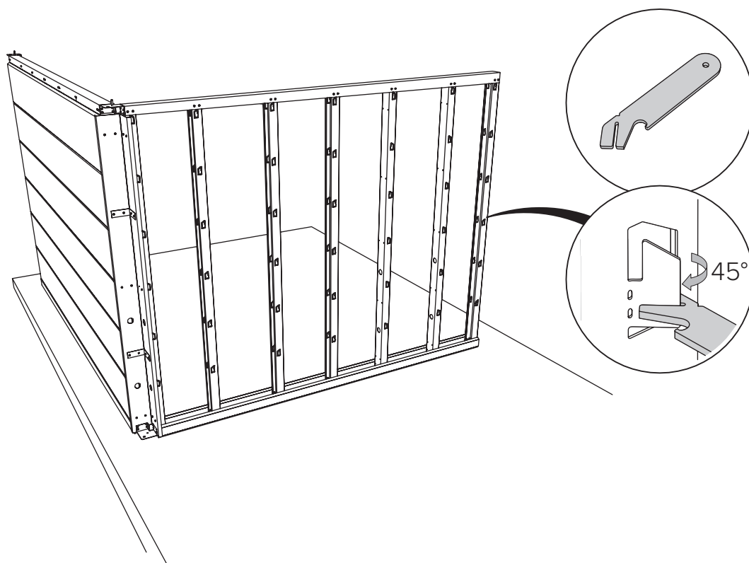
C + D Fachada / Fachada
