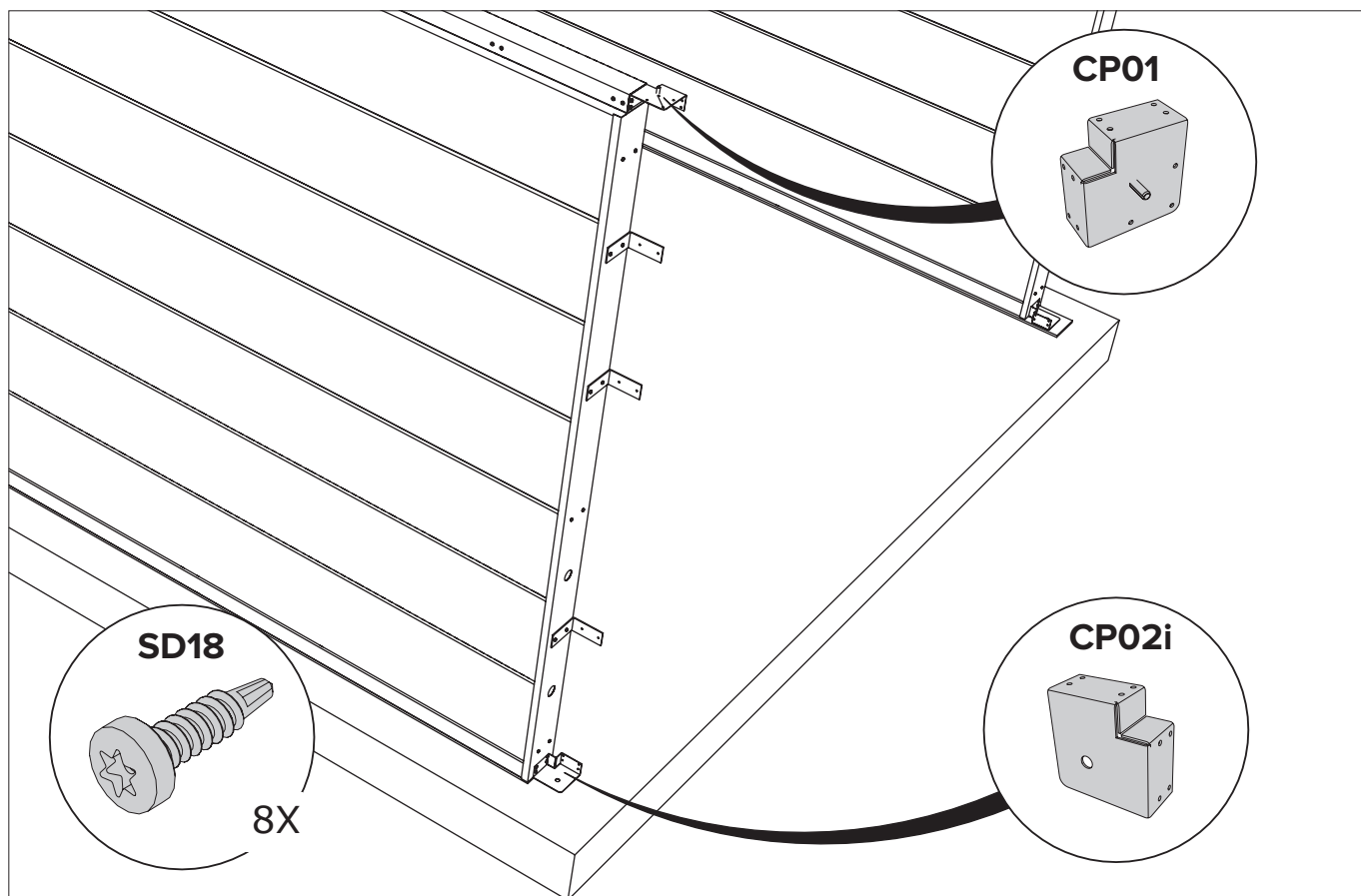
B1/B2/CD1/D2 Fachada / Fachada
