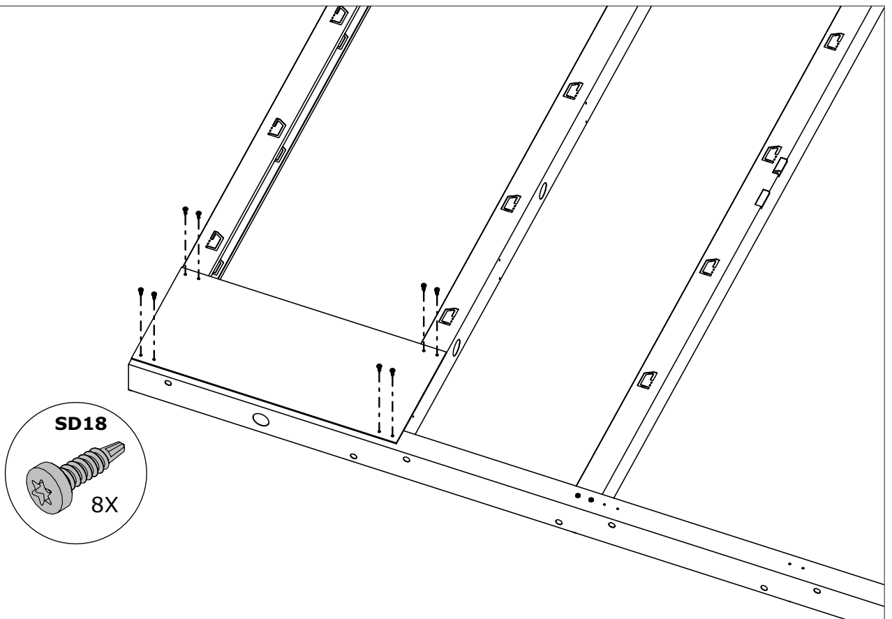
B2 Fachada / Fachada
