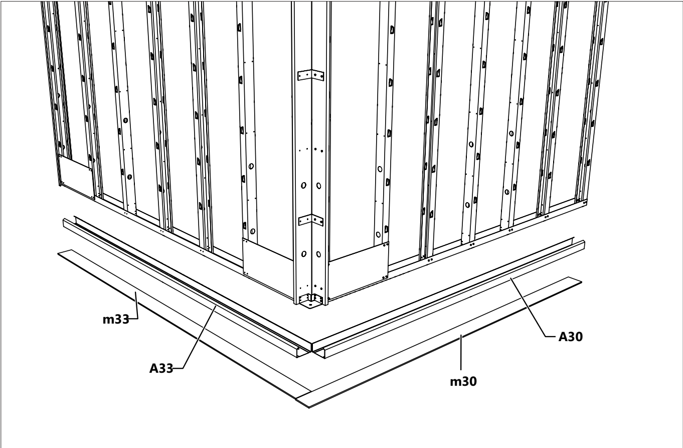
C/D1 Fachada / Fachada
