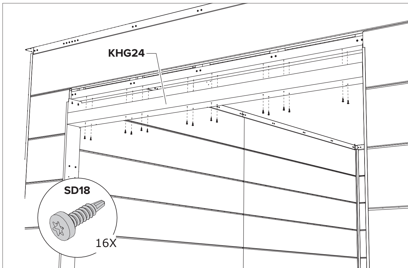
A Porta seccionada / Puerta seccional
