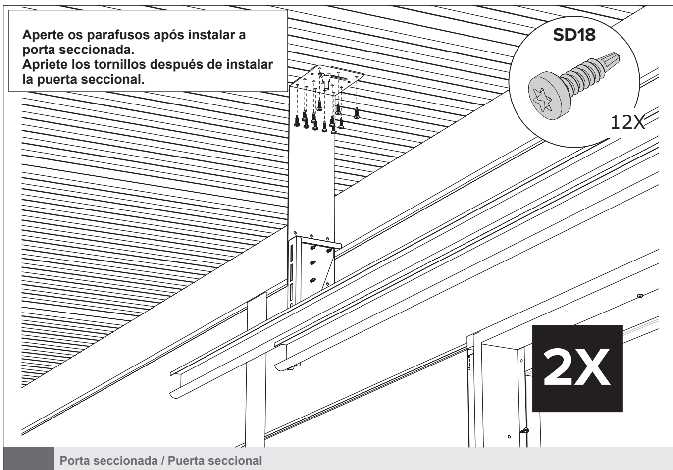
Porta seccionada / Puerta seccional
