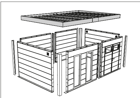
Cobertura / Cobertura
